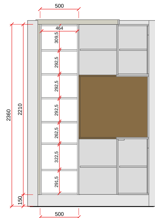
VISTA D - ESC. 1:30
