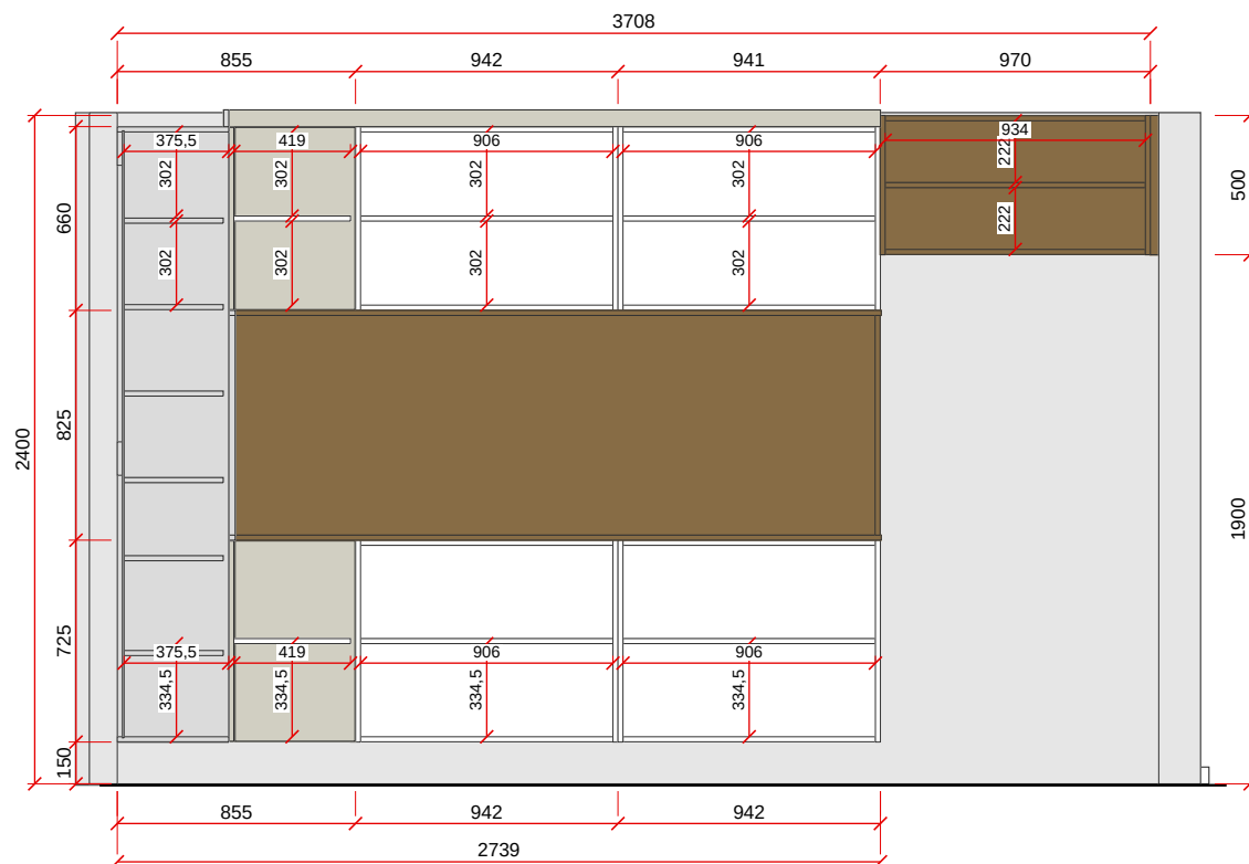
VISTA C - ESC. 1:30
