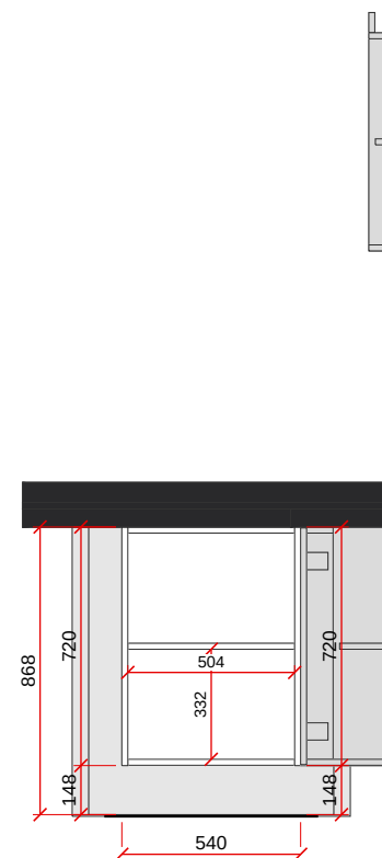
VISTA B - ESC. 1:25
