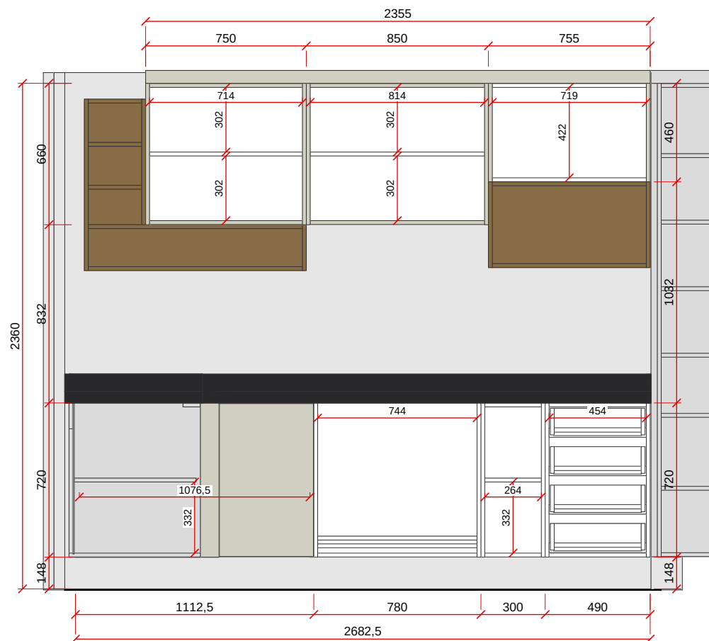
VISTA A - ESC. 1:25
